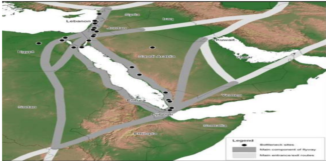
الشكل 2: خريطة للعناصر الرئيسية لممر الطيران في الوادي المتصدع/البحر الأحمر تبين مواقع الاختناقات الرئيسية (المصدر: المنظمة الدولية لحياة الطيور)
