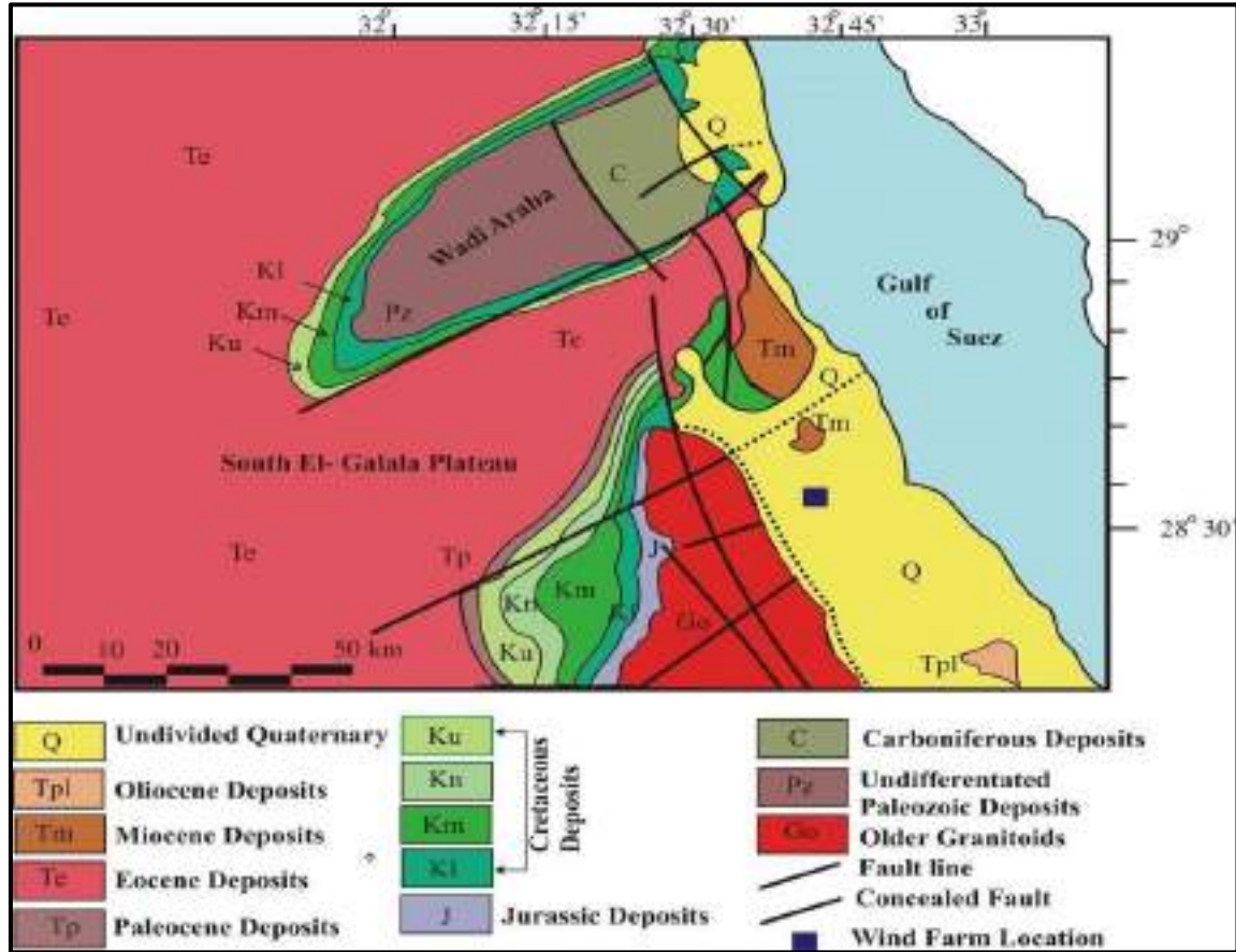
شكل رقم 30 الخريطة الجيولوجية الإقليمية للمنطقة المعدلة من الخريطة الجيولوجية لصخور القاعدة في مصر
