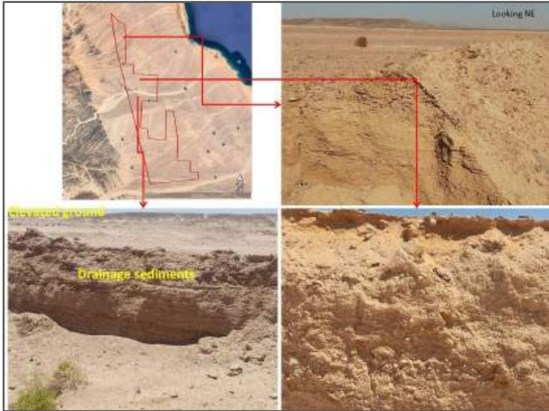
شكل رقم 36 الملمس والحالة الترسيبية لطبقة المصطبة ت2 في الجزء الشمالي من الموقع. لاحظ توزيع حجم الحبوب ودورات الترسيب لمصاطب الطبقة ت1
