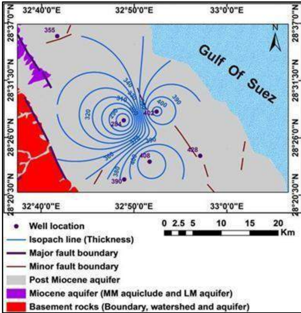
شكل رقم 38 خريطة توزيع سمك رواسب ما بعد الميوسين في حوض الحواشية، (مسعود وآخرون، 2012). لاحظ أن سمك الرواسب الرباعية (ما بعد الميوسين) يزداد باتجاه الشرق.
