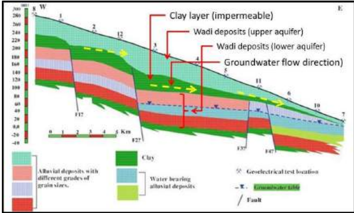
شكل رقم 40 مقطع عرضي كهرومائي على طول القناة الرئيسية لحوض دلتا وادي الحواشية يوضح طبقات سحنات رواسب ما بعد الميوسين (التقرير الداخلي لمركز التعافي من الكوارث 2001 في مسعود، 2012).
