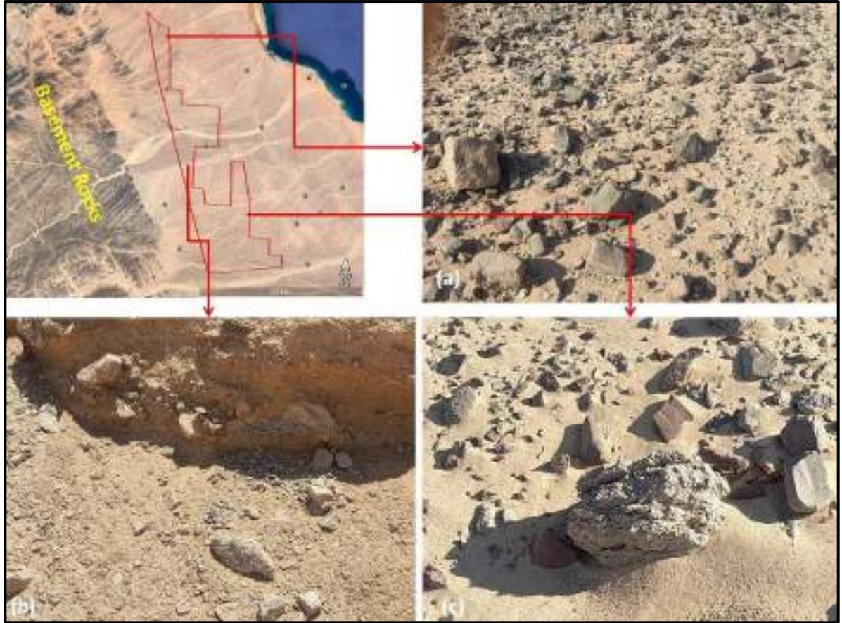
شكل رقم 31 القمم العالية لصخور القاعدة إلى الغرب من الموقع. تشكل الصخور شديدة التجوية من الجرانيت الأقدم (اللون الفاتح) والجرانيت الأصغر (اللون الداكن) بالإضافة إلى بعض شظايا البازلت من السدود الأساسية المتطفلة عبر صخور القاعدة
