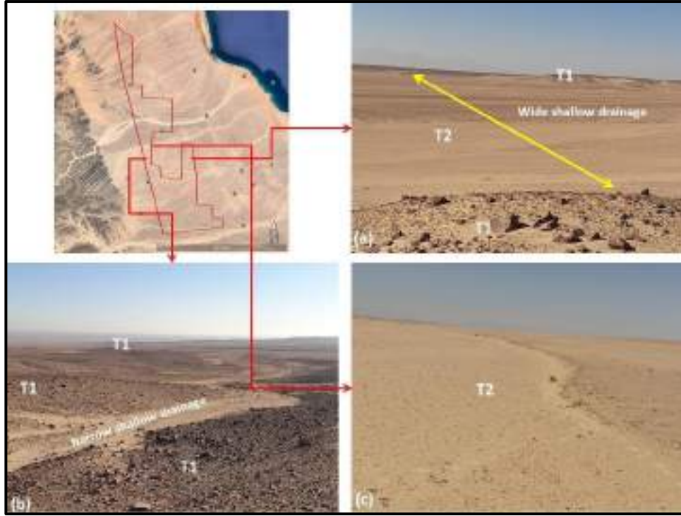
شكل رقم 34 ت1 وت2، (أ و ب) في الجزء الأوسط، و(ج) في الجزء الشرقي.
