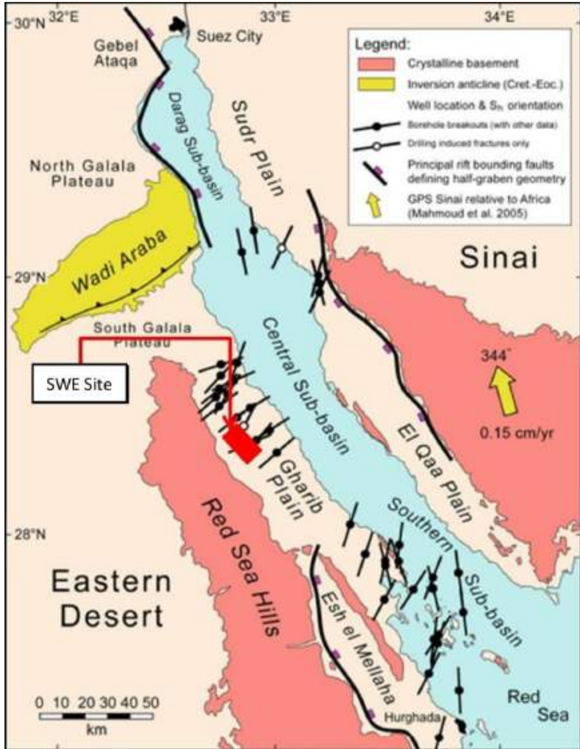
شكل رقم 29 المناطق الهيكلية لخليج السويس. يقع المشروع في سهل غريب. (بوسورث ودوروتشر 2017).
