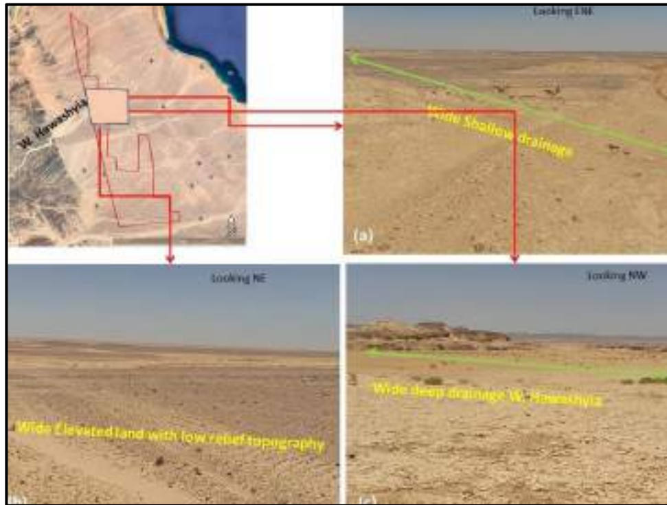
شكل رقم 25 مناطق النقش البسيط إما على طول خطوط الصرف الضحلة الواسعة (أ) أو سطح الأراضي المرتفعة. (ب) لاحظ أن التضاريس الوعرة في الجزء العلوي من وادي الحواشية (ج)
