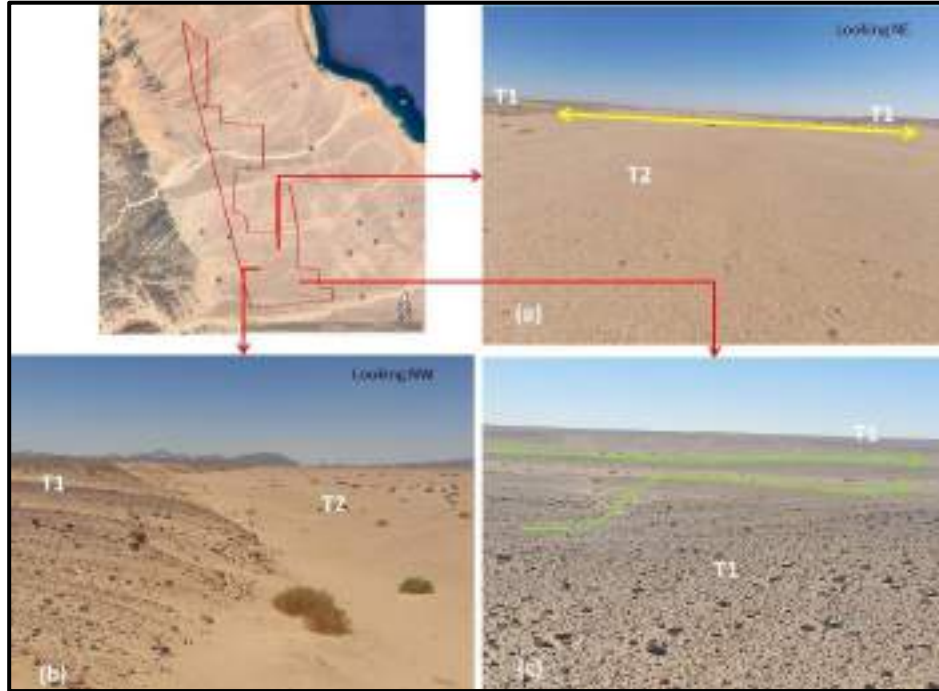
شكل رقم 35 طبقة المصطبة 1 والمصطبة 2 في الجزء الجنوبي من الموقع. يرجى العلم أن نسيج مظهر الطبقة ت1 (حجم الحبيبات الخشنة جدًا) وت1 (الحبيبات الناعمة)
