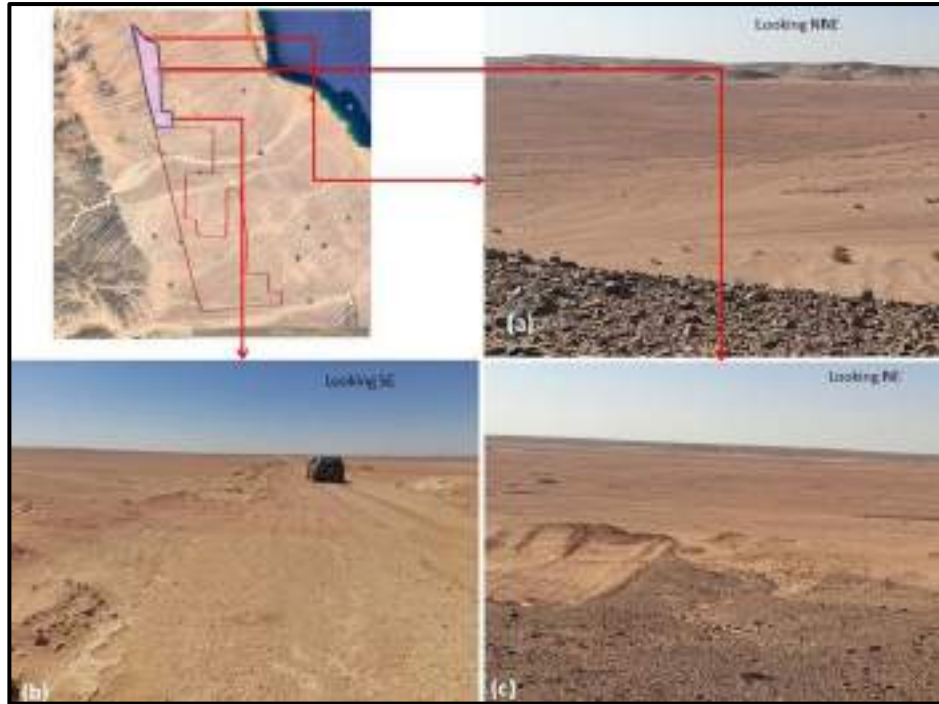
شكل رقم 24 التضاريس الطبيعية لموقع المشروع. خطوط تصريف واسعة وضحلة تحدها أراض مرتفعة.
