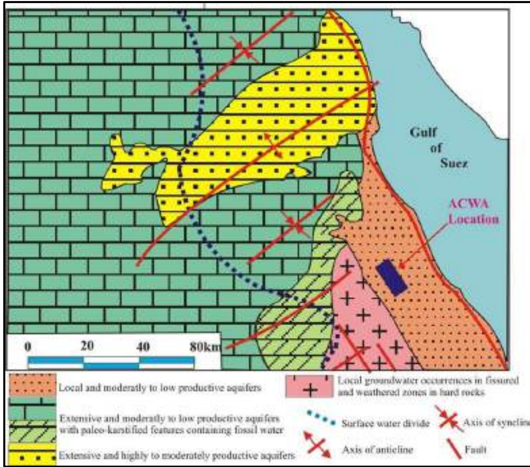
شكل رقم 39 الخريطة الهيدروجيولوجية للمنطقة المحيطة بموقع المشروع.
