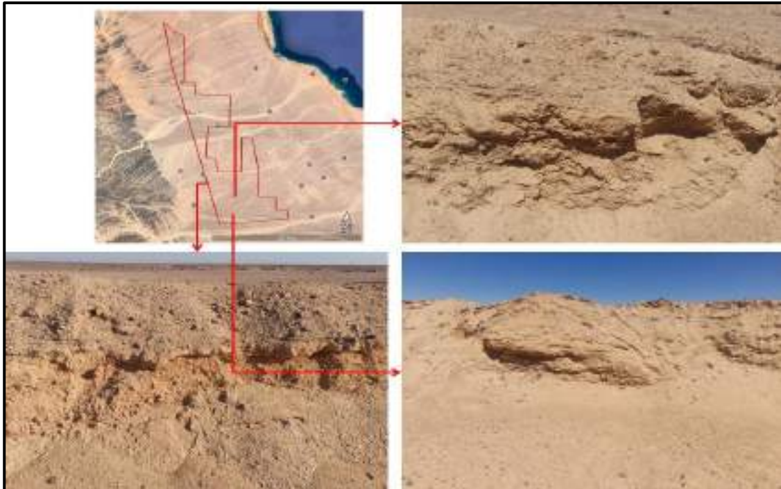
شكل رقم 37 نسيج وحالة ترسب طبقة المصطبة ت2 في الجزء الأوسط من الموقع. لاحظ توزيع حجم الحبيبات ودورات الترسيب في المصاطب ت1.
