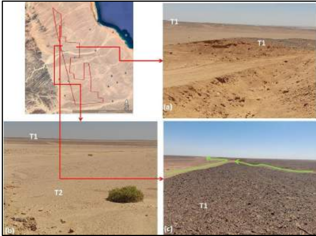
شكل رقم 33 المصطبة ت1 والمصطبة ت2 في الجزء الأوسط من الموقع. يرجى العلم أن السطح المتقارب حجم الحبيبات للمصطبة ت1 يحمل معه بسبب تدفق المياه السطحية والرياح رواسب دقيقة إلى المصطبة المنخفضة ت2، (ب)
