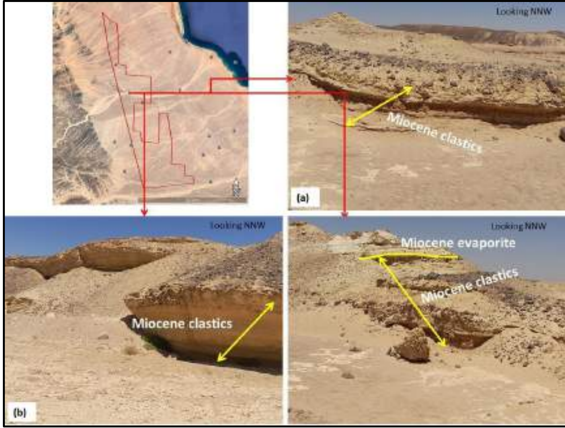
شكل رقم 32 طبقات الصخور الفتاتية من الميوسين السفلي تغطي الطبقات السفلية.
