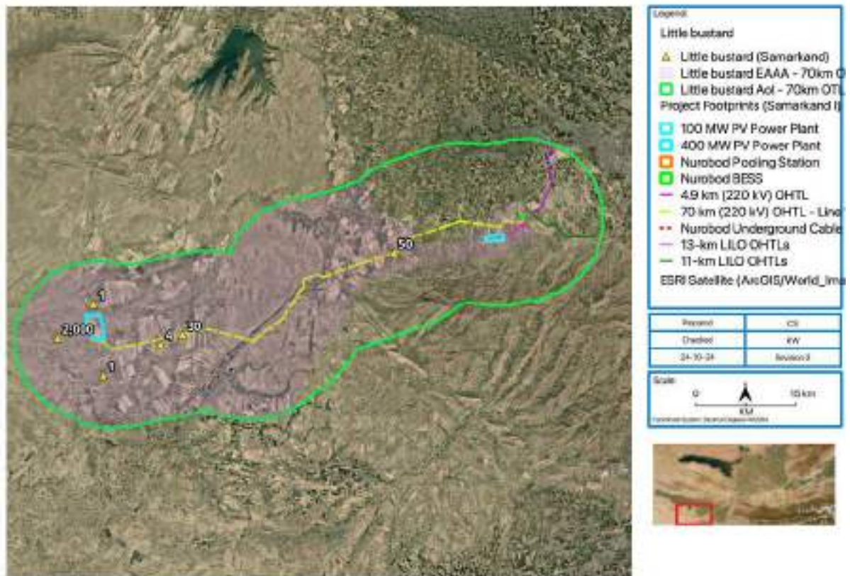
Рисунок 5-1 Критическое место обитания стрекета (малой дрофы) по отношению к фотоэлектрической станции мощностью 400 МВт и 70-километровой зоне ВЛЭП в Нурабадском районе
