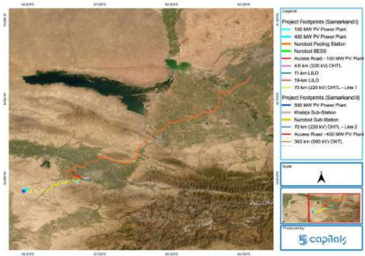
Рисунок 2-7 Прилегающие, планируемые объекты генерации, хранения и передачи электроэнергии, входящие в состав Проекта и связанного с ним Проекта Самарканд II Солнечная фотоэлектрическая станция и АСХЭ
