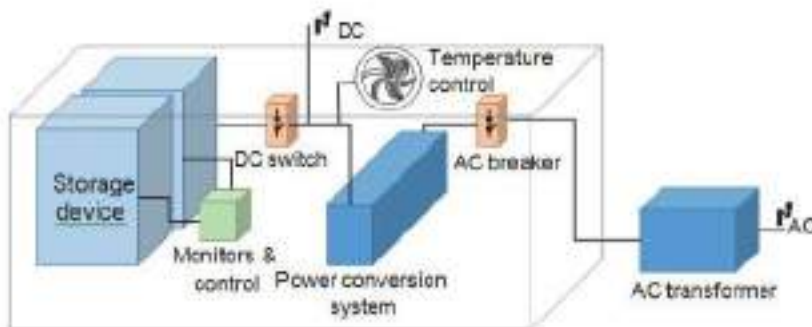
Рис. 2-5 Общая схема системы АСХЭ
